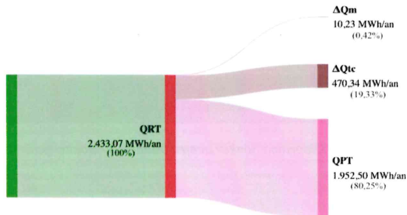
Figura 12.3 – Diagrama Sankey pentru bilanțul termoeenergetic real al RT – sezonul de vară
