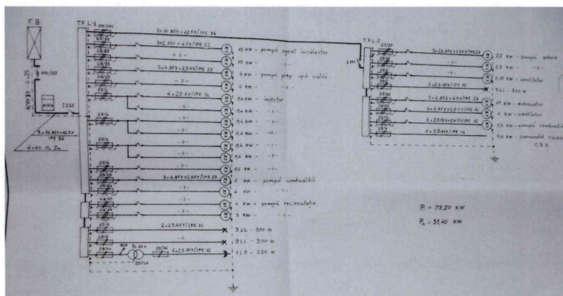
Figura 6.2 – Schema electrică monofilară pentru CT Florilor – Nord și Sud
