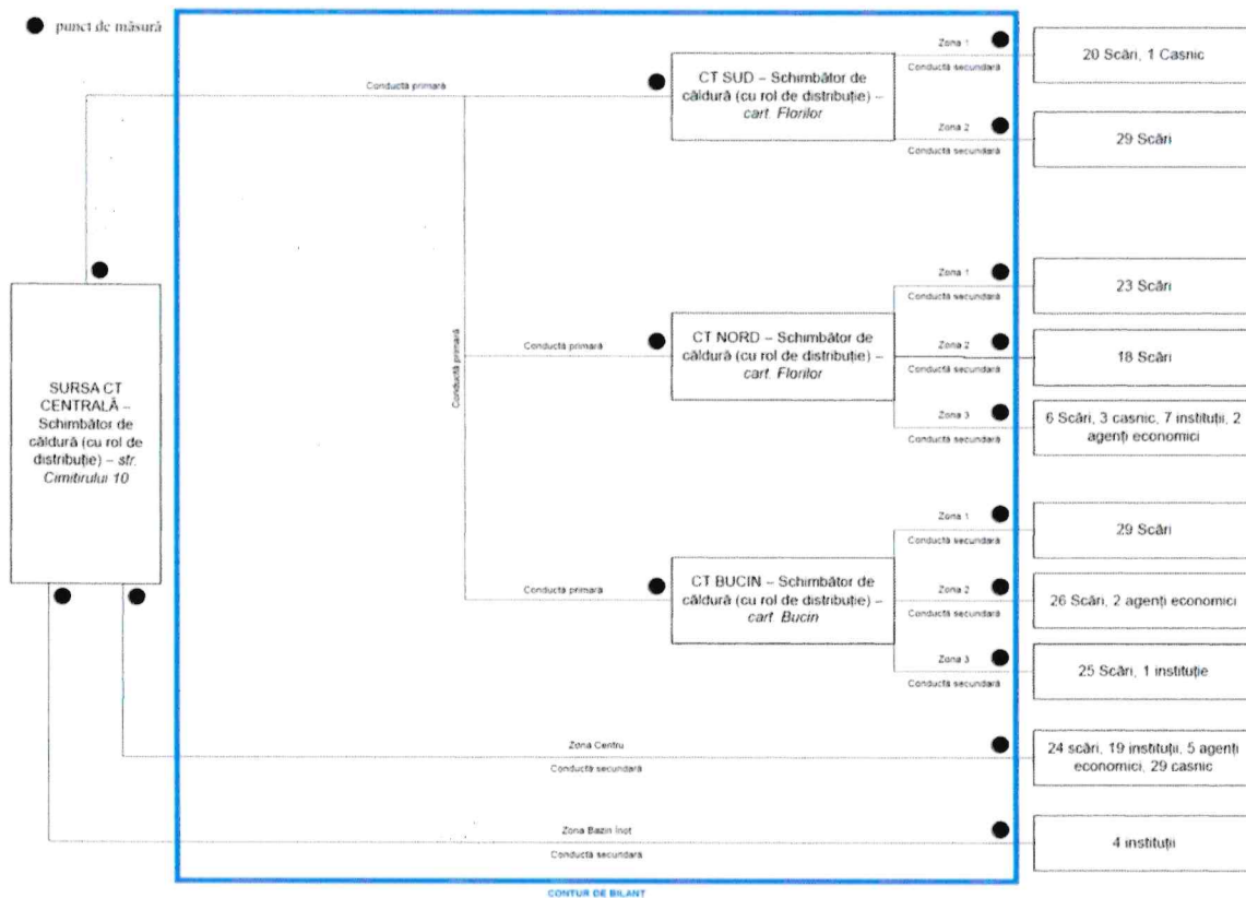
Figura 9.1 – Schema fluxului tehnologic al SACET Gheorgheni și punctele de măsură
