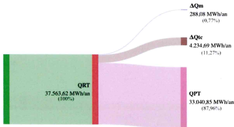
Figura 12.1 – Diagrama Sankey pentru bilanțul termoeenergetic real, anual, al RT
