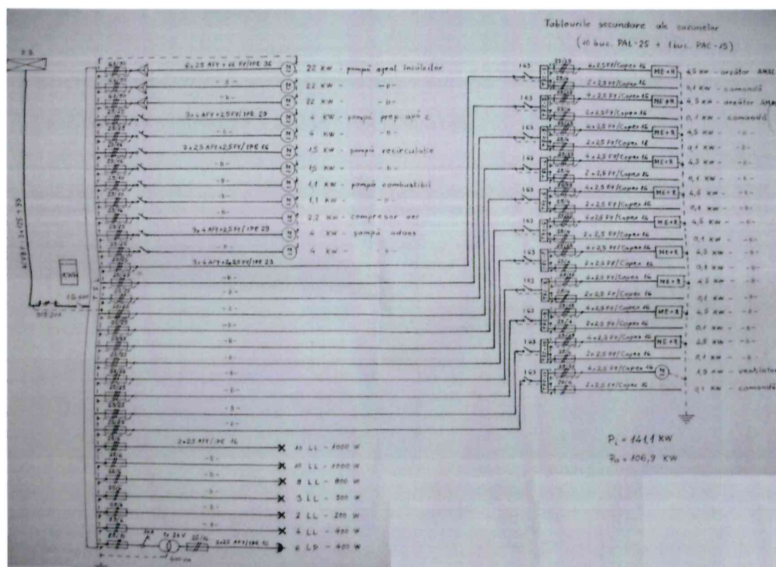
Figura 6.4 – Schema electrică monofilară a CT Bucin
