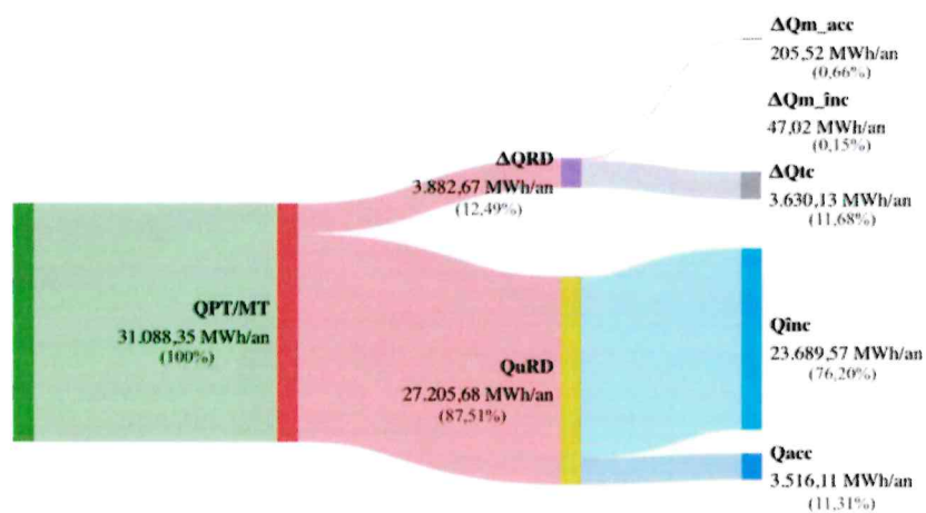
Figura 12.6 – Diagrama Sankey pentru bilanțul termoeenergetic real al RD – sezonul de iarnă
