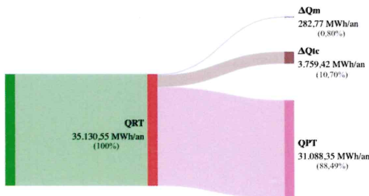
Figura 12.5 – Diagrama Sankey pentru bilanțul termoeenergetic real al RT – sezonul de iarnă
