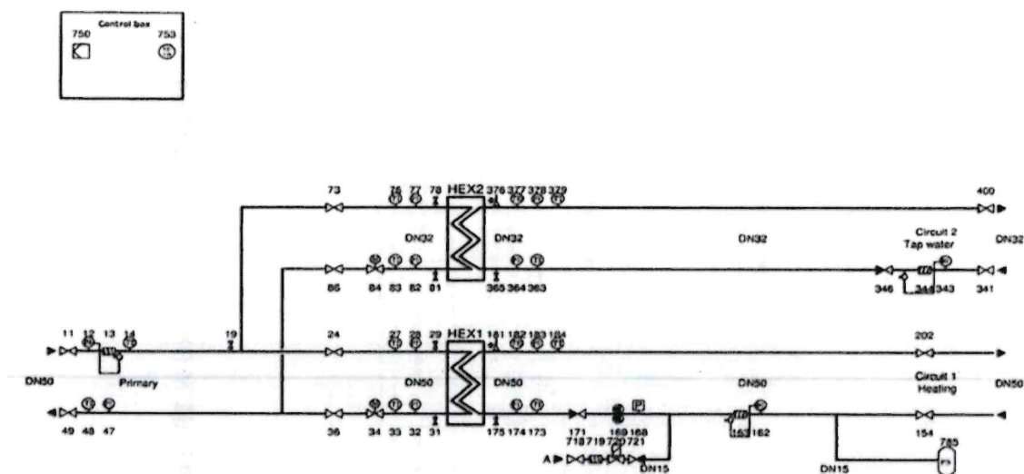
Figura 4.5 – Schema tehnologică a modulelor termice
