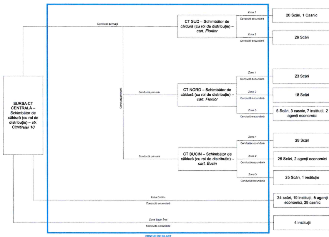
Figura 5.1 – Schema simplificată a SACET Gheorgheni
