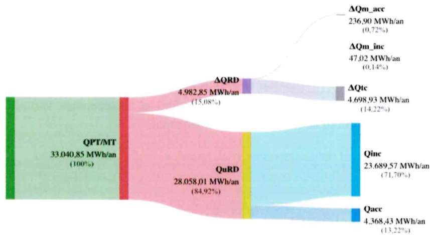
Figura 12.2 – Diagrama Sankey pentru bilanțul termoeenergetic real, anual, al RD
