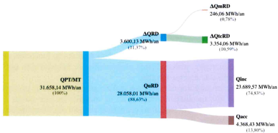
Figura 17.2 - Diagrama Sankey – bilanțul optimizat al rețelei de distribuție
