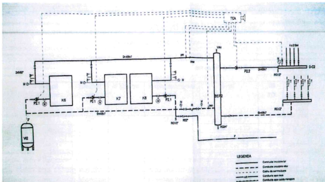
Figura 4.4 – Schema tehnologică a CT Bucin
