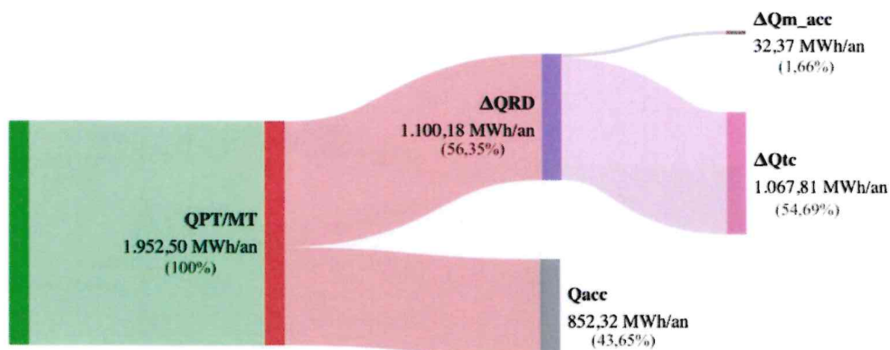
Figura 12.4 – Diagrama Sankey pentru bilanțul termoeenergetic real al RD – sezonul de vară
