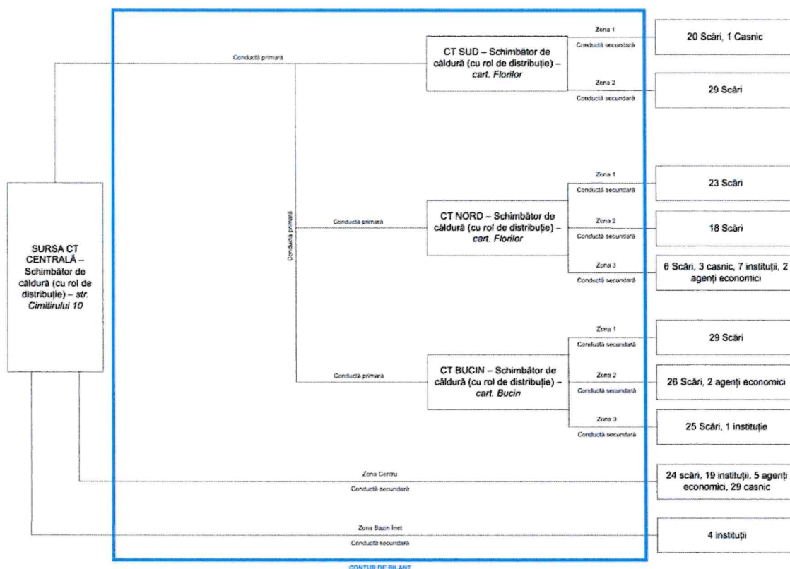
Figura 4.1 – Schema tehnologică a SACET Gheorgheni
