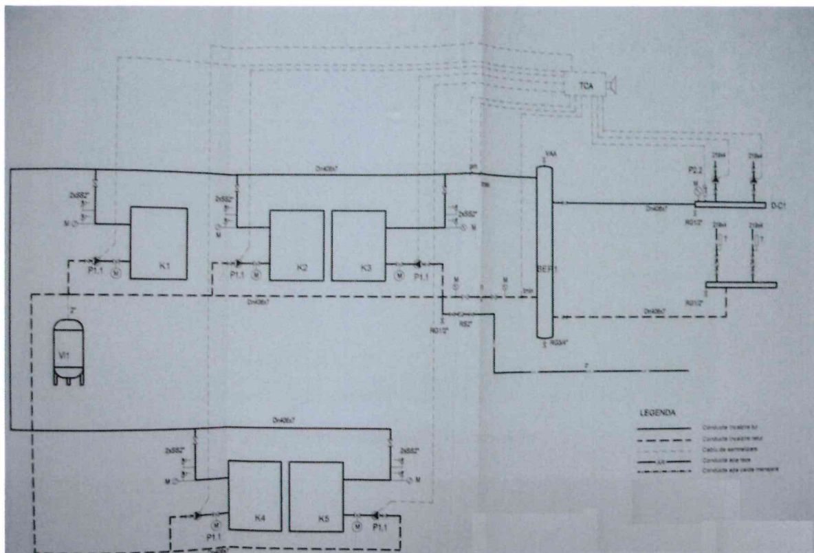
Figura 6.1 – Schema tehnologică pentru CT Florilor – Nord și Sud
