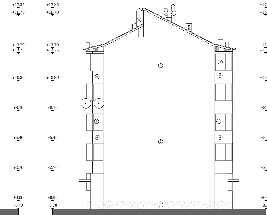
FATADA SUD EXISTENTA
