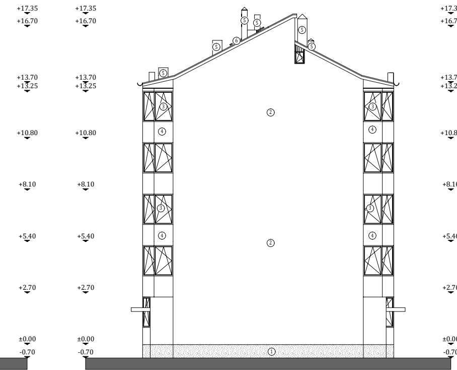
FATADA SUD PROPUSA
